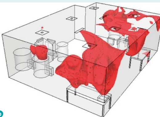
Les points représentés sont ceux avec un âge de l'air de 160 secondes. a. design 1 ; b. design 2.
