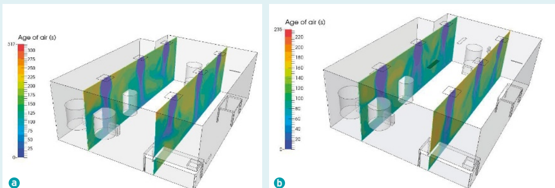
a. design 1 ; b. design 2.
