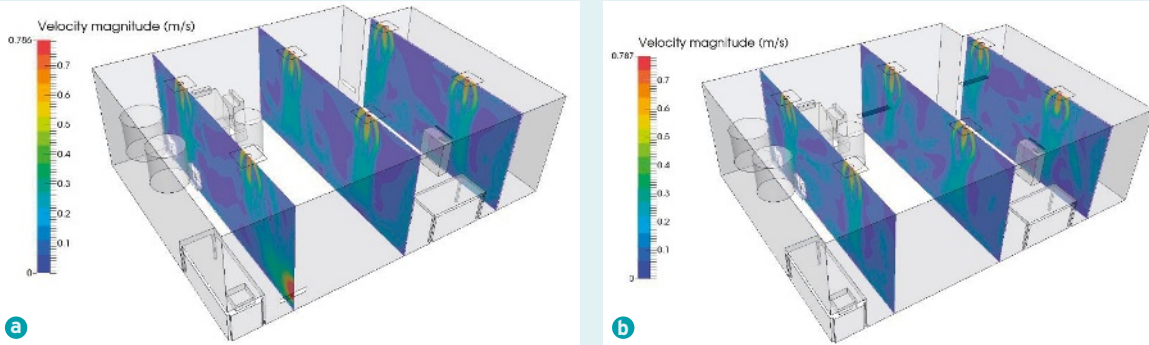
a. design 1 ; b. design 2.
