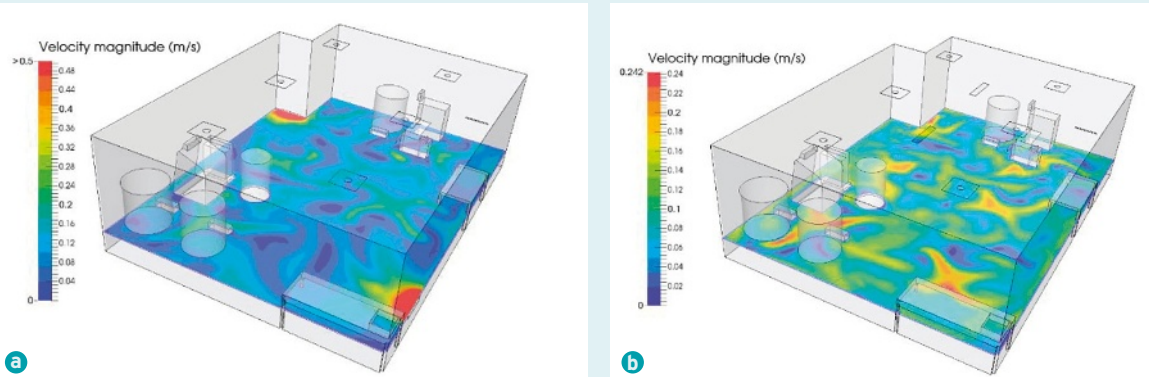
a. design 1 ; b. design 2.
