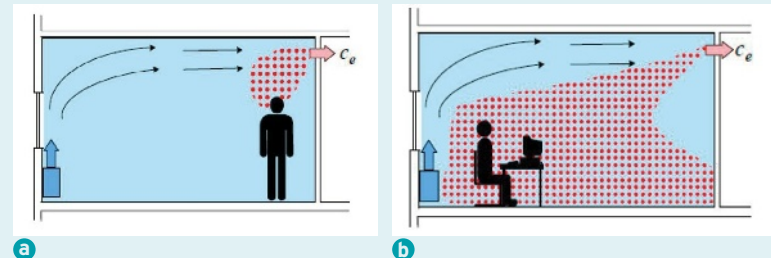
a. la source de contamination est proche de la reprise et la concentration moyenne dans la pièce est faible ; b. la concentration moyenne dans la pièce est élevée.
