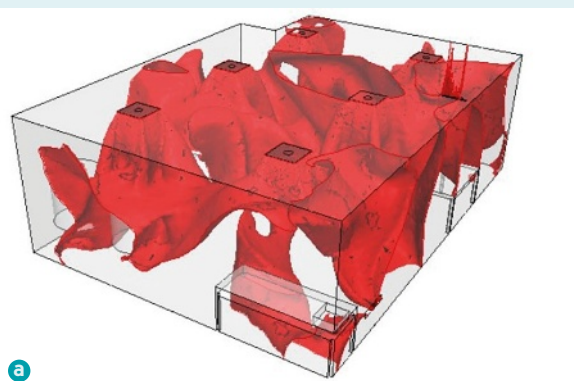
Les points représentés sont ceux avec un âge de l'air de 160 secondes. a. design 1 ; b. design 2.
