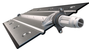
MESURE DE PRESSION DIFFÉRENTIELLE VIA LE CLAPET DE RÉGULATION
